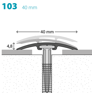
D.O.S. overgangsprofiel Aluminium. Voor vloerhoogtes 0-17,5 mm.
