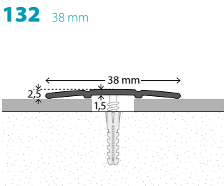
Overgangsprofiel Aluminium. Centraal geboord
