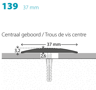
Versterkt overgangsprofiel Aluminium.
