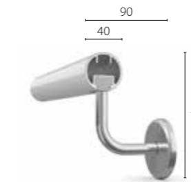
HREB-6-S75
