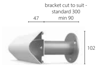
BL-10HE
