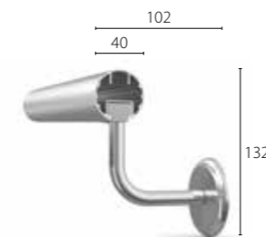
HRA-6-S87
