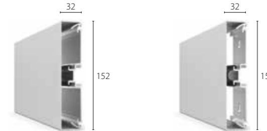
SCR-150MN
