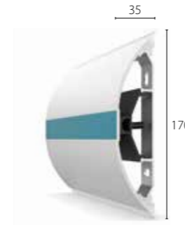
SCR-170
