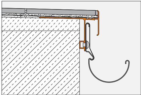
Mise en œuvre du Schlüter-DITRA avec Schlüter-BARA-RTKEG
