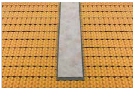
Étanchéification des raccords avec Schlüter®-KERDI-KEBA
